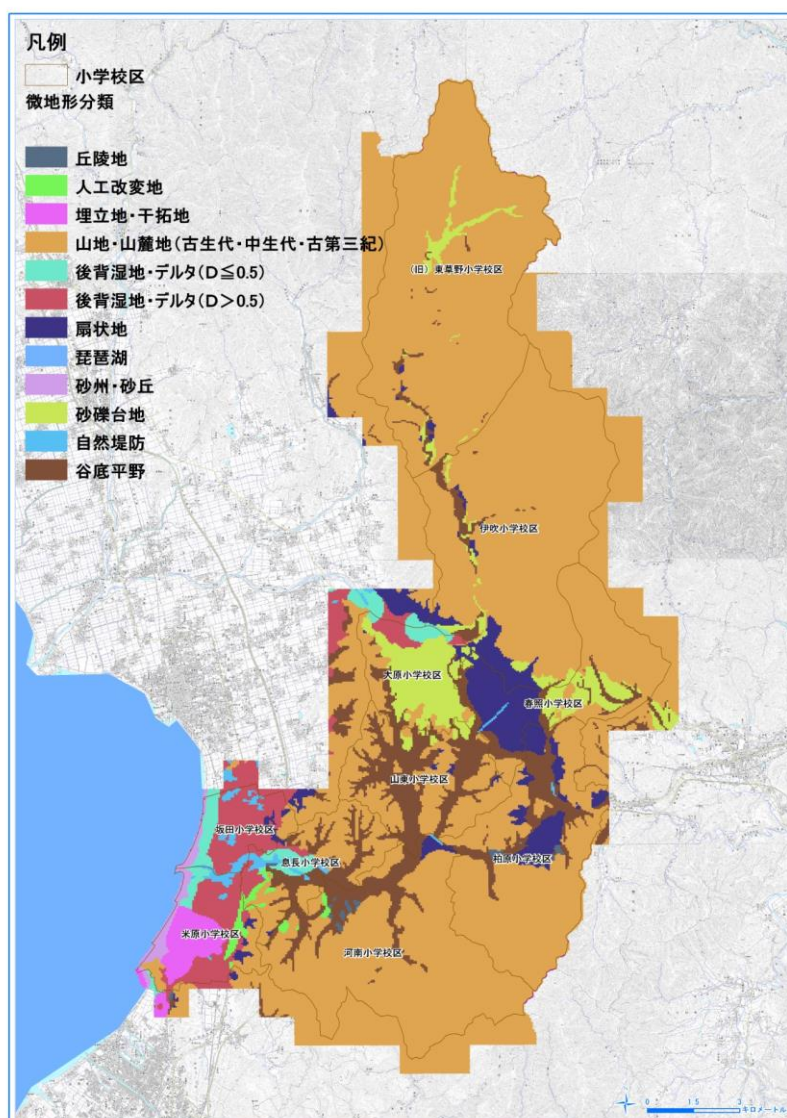
米原市の地形分類図
