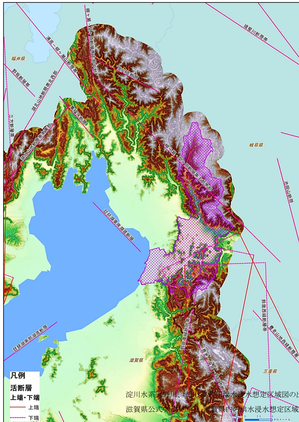
本市周辺の活断層位置図
