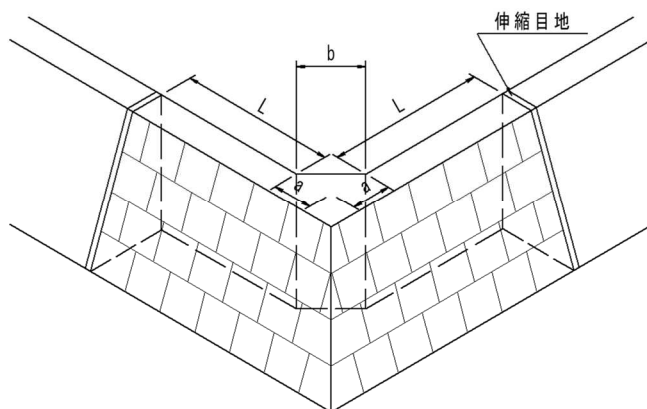
(a) 立体図
