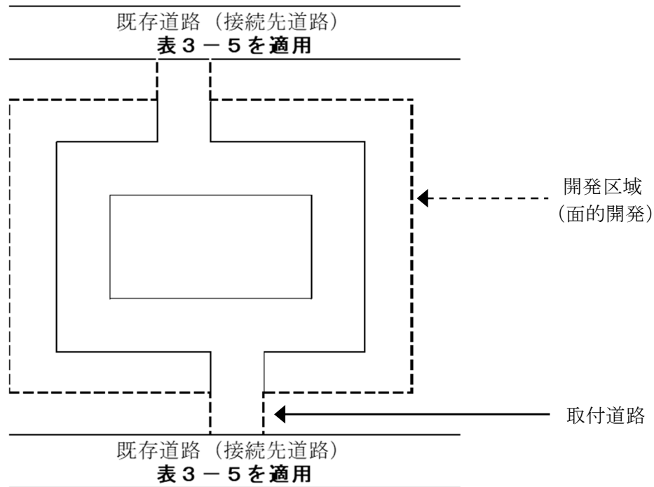
図 3 - 5 接続先道路
