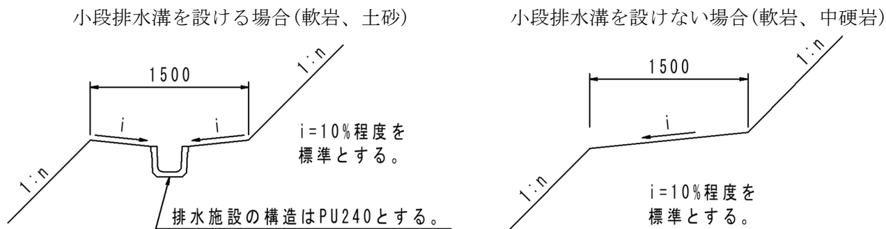
図 11-2 切土の小段
