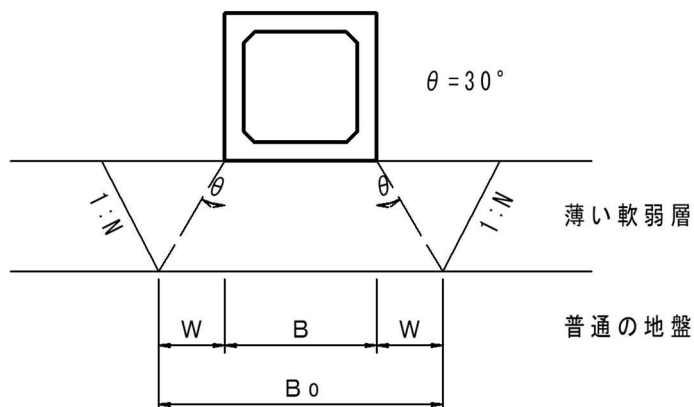
図 3-13 置換基礎
