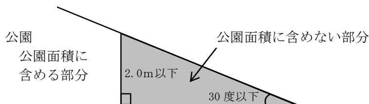
図4-1 公園面積に含めない部分（隅部）
