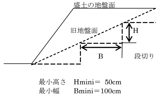
図 11-6 段切り
