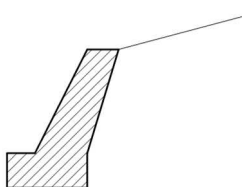
図 11-13 擁壁の自重
