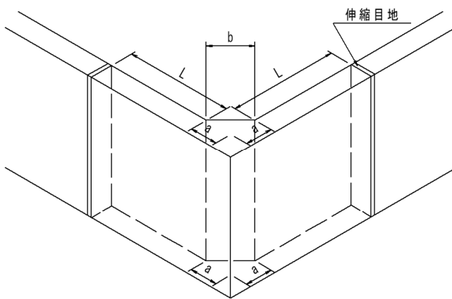
(a) 立体図
