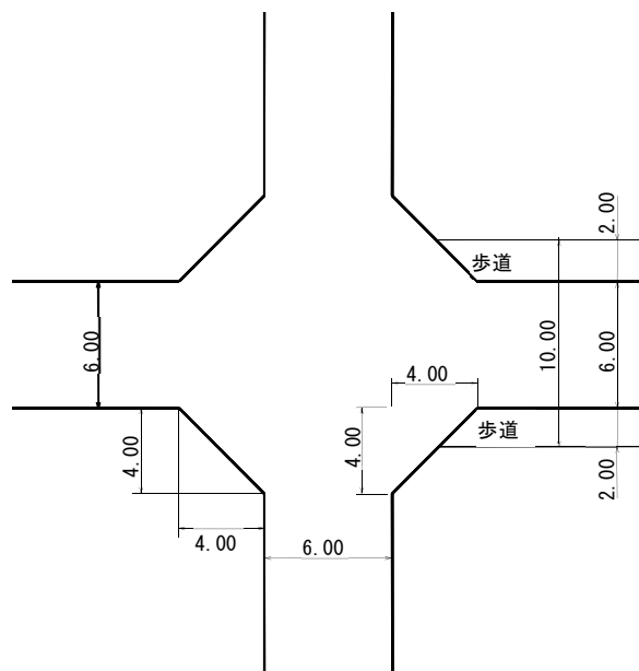
図 3-9 隅切り設計図
