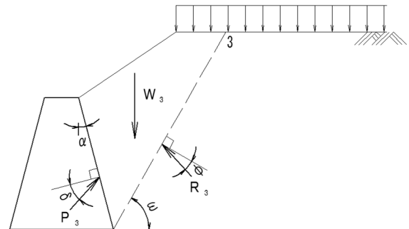
②仮定されたくさび (すべり線位置 3)
