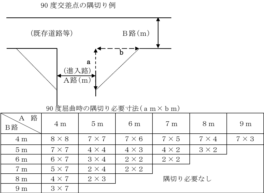
別図1 道路隅切り図
