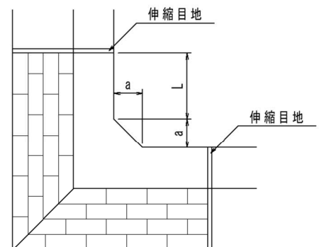
(b) 平面図
