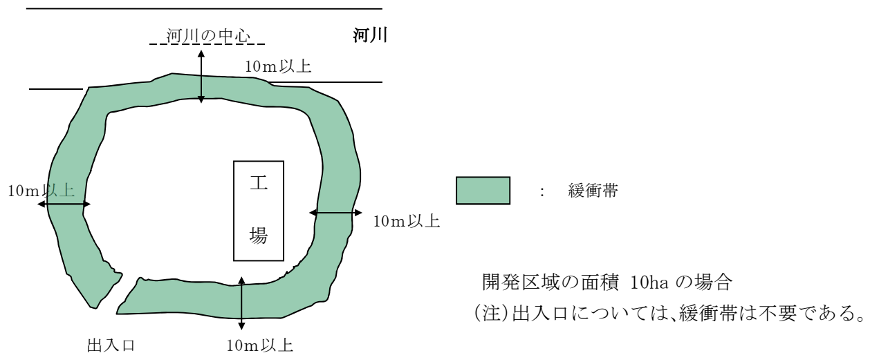
図 7－1 緩衝帯配置図
