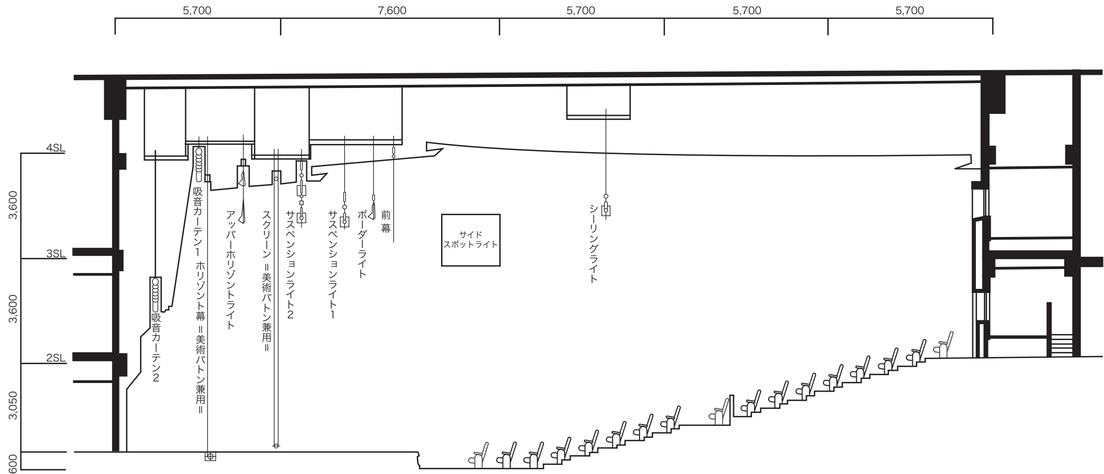
ベルホール310 舞台断面図
